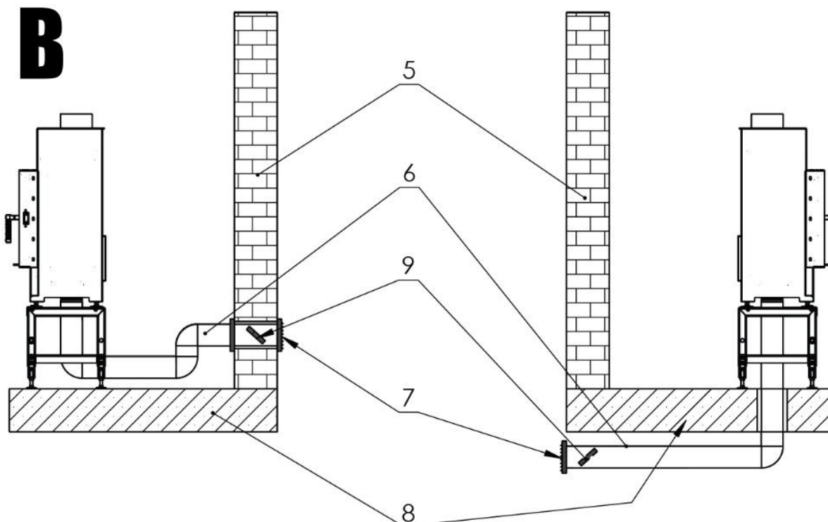
Rys. 3. [PL] Doprowadzenie powietrza/ [CZ] Přívod vzduchu/ [HU] Légbevezetés/ [SK] Prívod vzduchu/ [EN] Air supply/ [LT] Oro tiekimas/ [LV] Gaisa raideve/ [RU] Подача воздуха/ [EE] Õhuvarustus/ [GR] Παροχή αέρα/ [RO] Alimentarea cu aer/ [BG] Подаване на въздух/ [UA] Пoдaчa пoвiтря/ [NL] Luchttoevoer/ [HR] Dovod zraka/ [TR] Havanın beslenmesi/ [PT] Aporte de ar/ [FR] Arrivée d'air/ [ES] Suministro de aire
