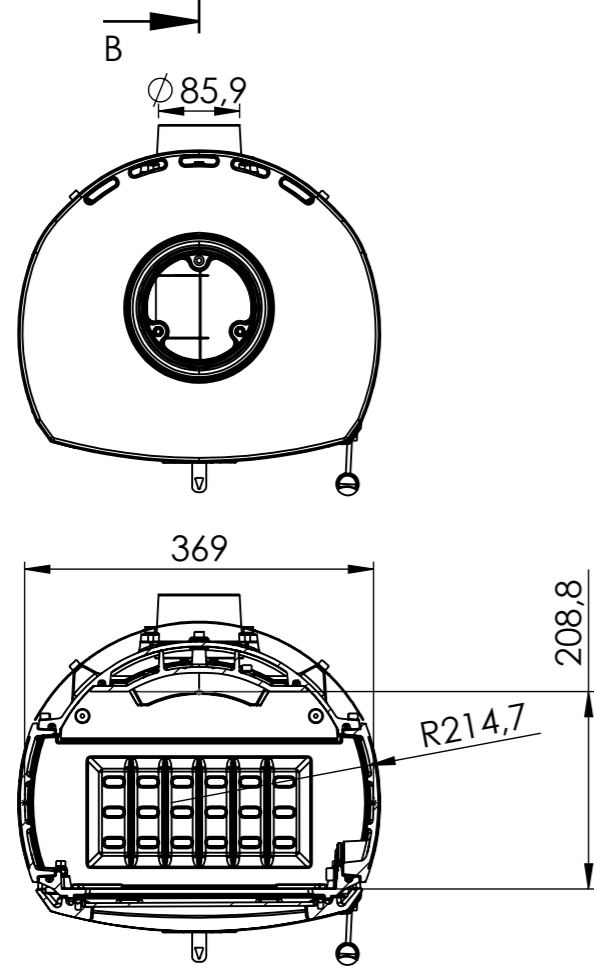
PRZEKRÓJ A-A
